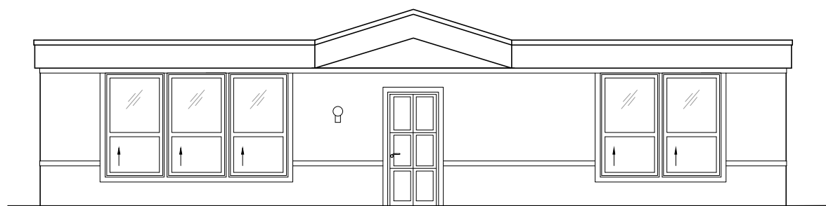
ELEVATION B
